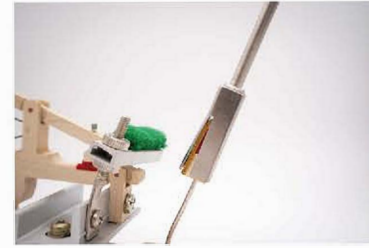
[G303] バックチェック 回し
