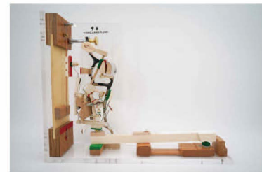
[G605] UP アクションモデル 1 鍵
