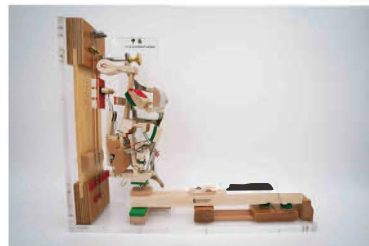
[G604] UP アクションモデル 2 鍵
