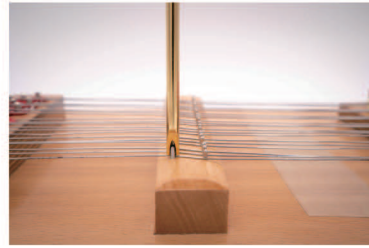
[G501] 駒ピン打ち下ろし
