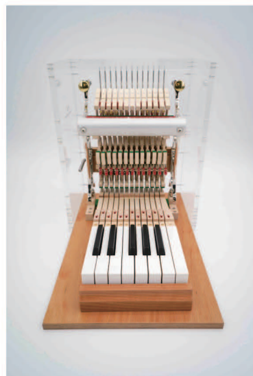
[G606] UP アクションモデル 13 鍵 受注生産
