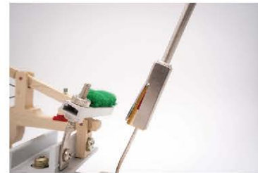
[G303] バックチェック 回し 価格：1,980 円 (税込み)
